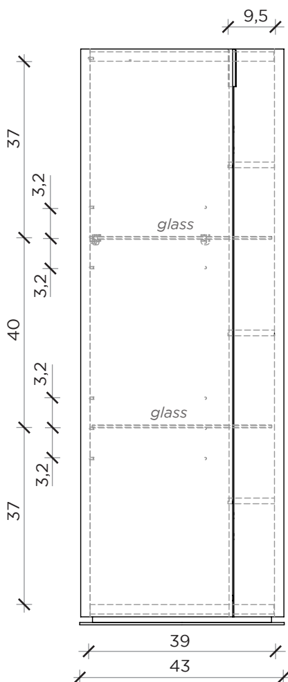
LATO | SIDE
