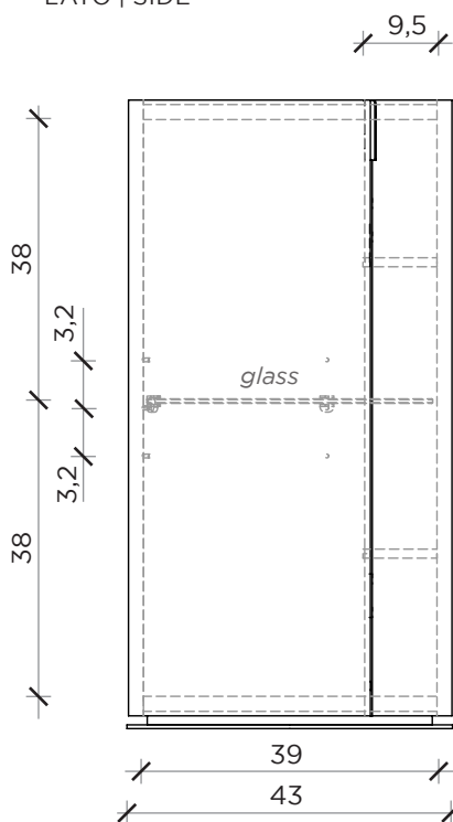
LATO | SIDE
